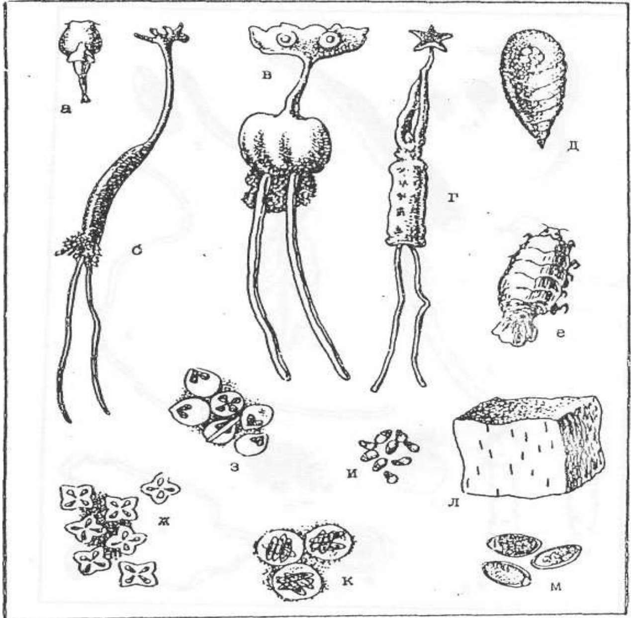
Рисунок 1: а-е паразитические ракообразные (а - Калигус, б - Пинелла, в - Офирион, г - Псевдотрахелиастес, д - Саркотацес, е - Изопода; длина от 0,5 до 15 см); ж-л - паразитические простейшие (ж-к - споры и ооцисты под большим увеличением микроскопа; л - цисты микроспоридий или микроспоридий в кусочке мышечной ткани - примерно натуральная величина); м - яйца трематод под большим увеличением микроскопа.
